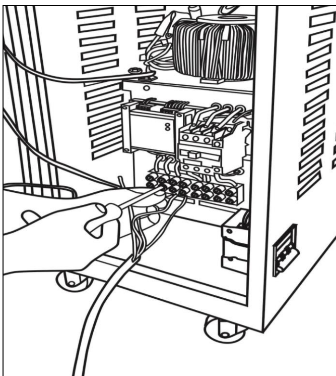
Рис. 3. Подключение нагрузки к клеммной колодке
