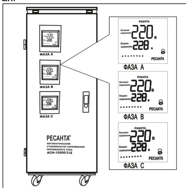
Рис.9. Показания дисплея после включения
