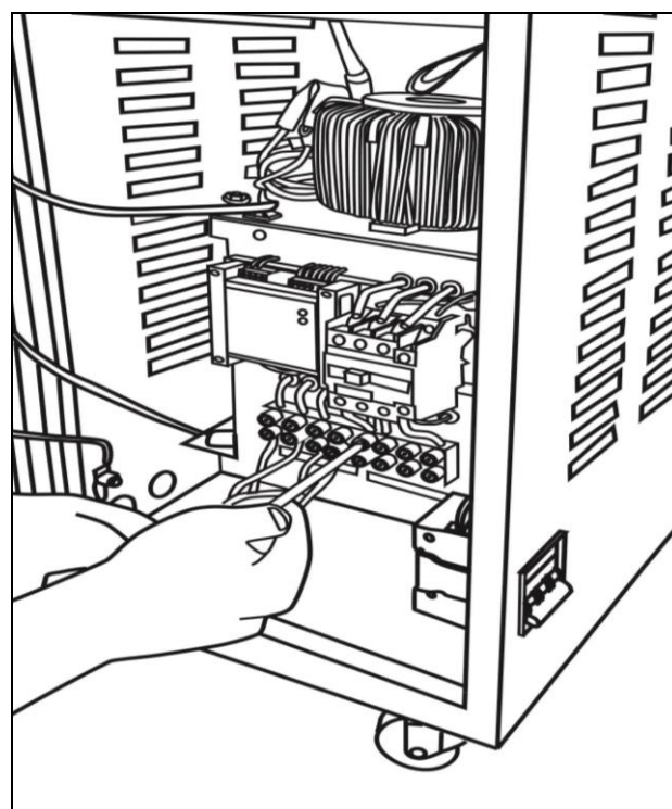
Рис. 4. Проверка протяжки всех болтов клеммной колодки
