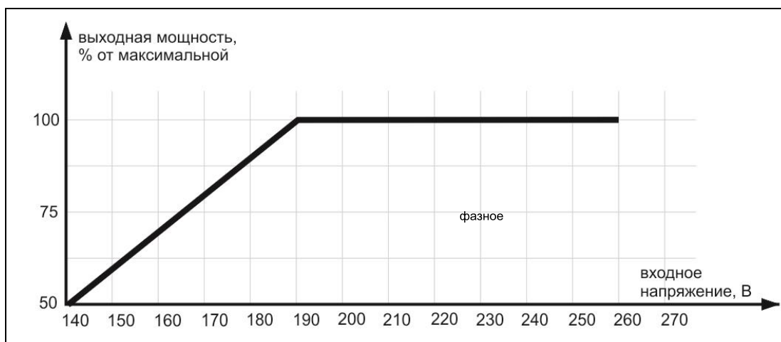
Рис. 2. График зависимости выходной мощности стабилизатора от входного напряжения для каждой фазы.
