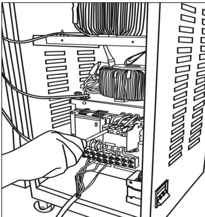
Рис 5. Протяжка болтов контактора
