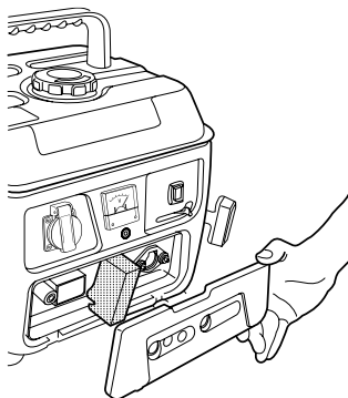
Фильтрующий элемент
